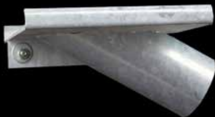
Kabelausslass 30° Ø 70 mm ARCOSYSTEM® Größe 1 Art.-Nr. VT1011-P002-A019
